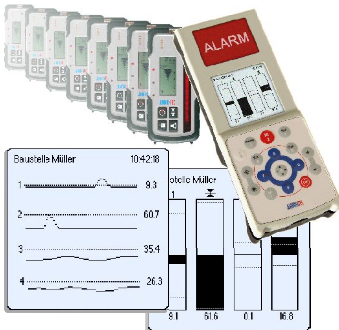
Bildschirmdarstellungen bei Verwendung von 4 Metor-RF Laserdetektoren
